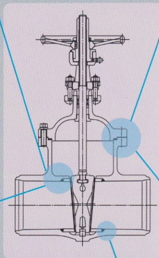
小判胴型のガスケット面修正加工
