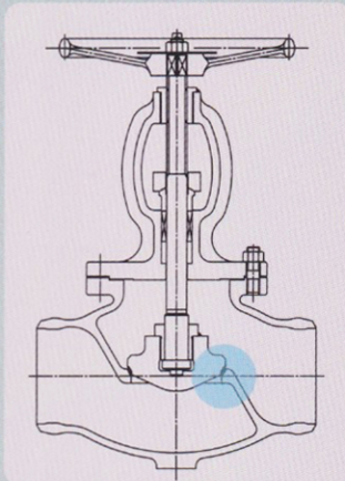
玉形弁
