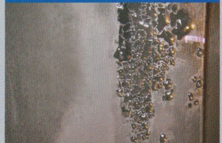
自動溶接によるシートリング接続部のエロージョン部分肉盛
