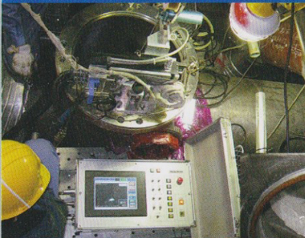
新しいシートリングの溶接
